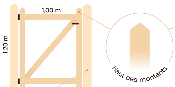
Poteaux 12 x 12 de Classe 4 pour une stabilité maximale
